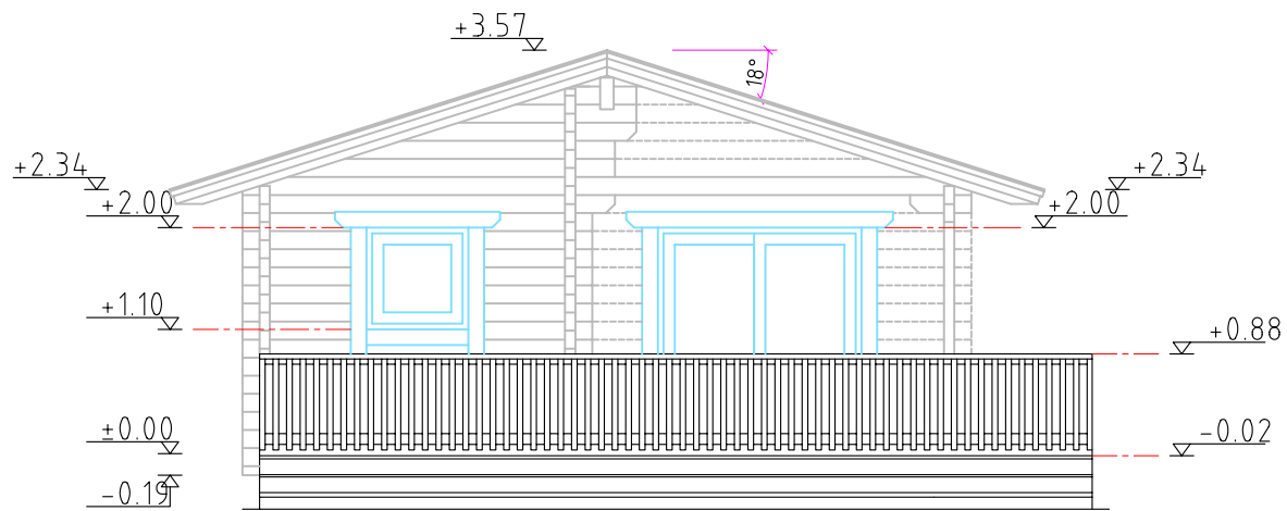
Elevation - C
