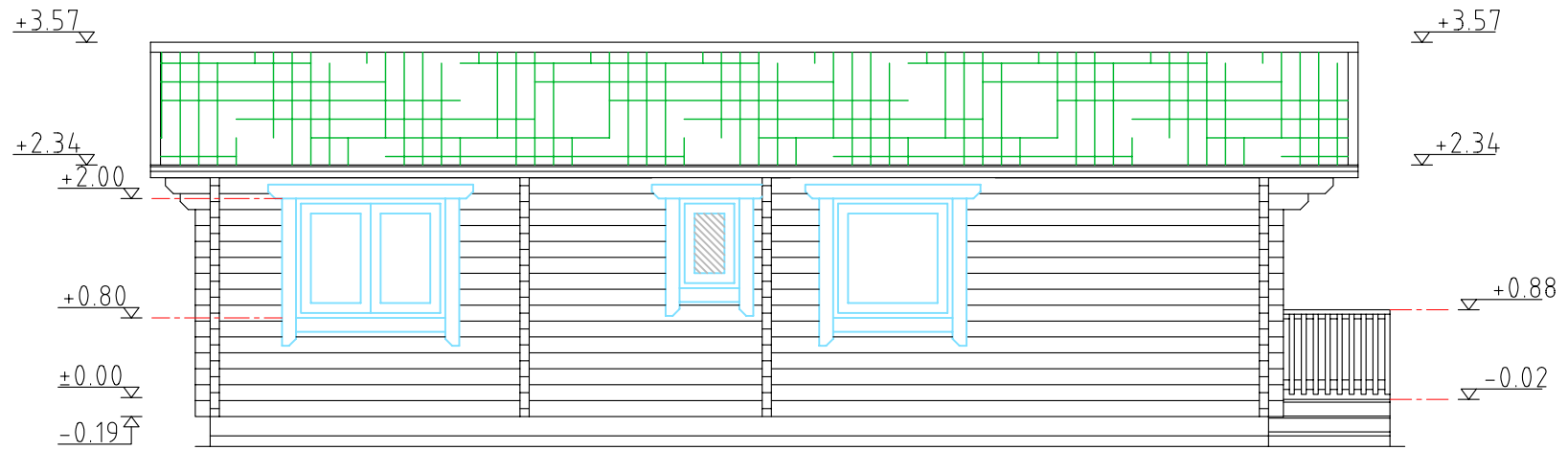
Elevation - B
