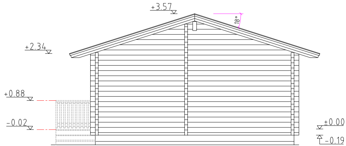
Elevation - D
