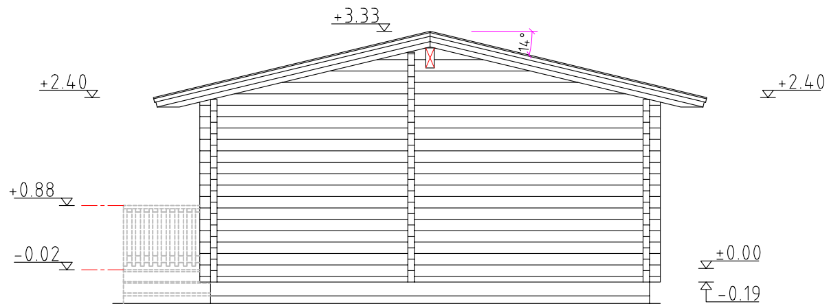
Elevation - D
