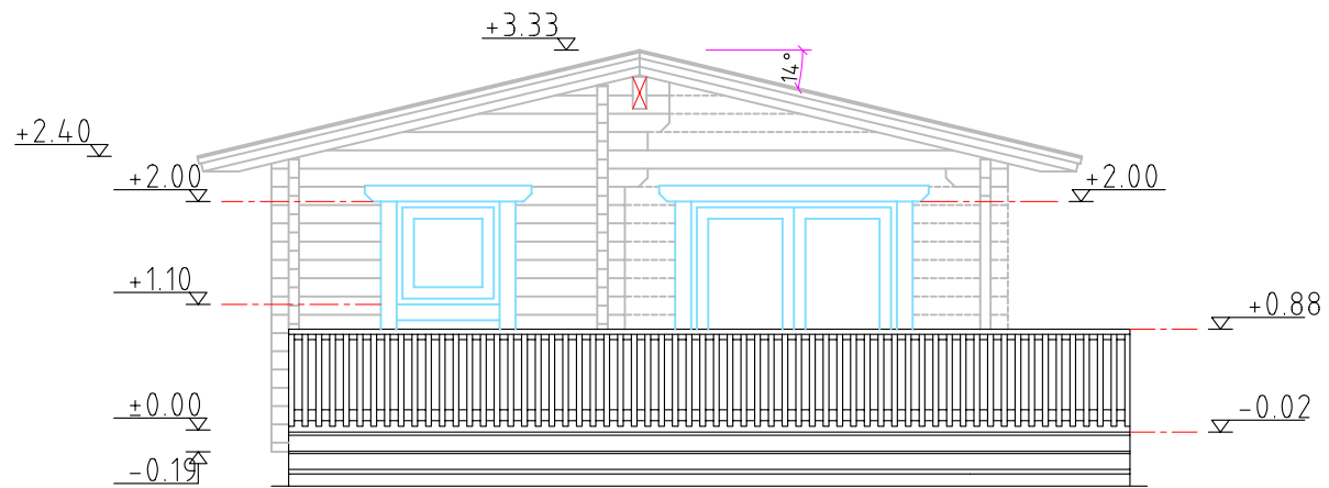
Elevation - C
